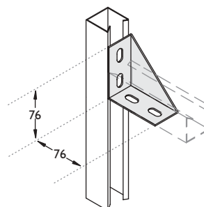
Cantoneira Reforçada com 4 Furos
